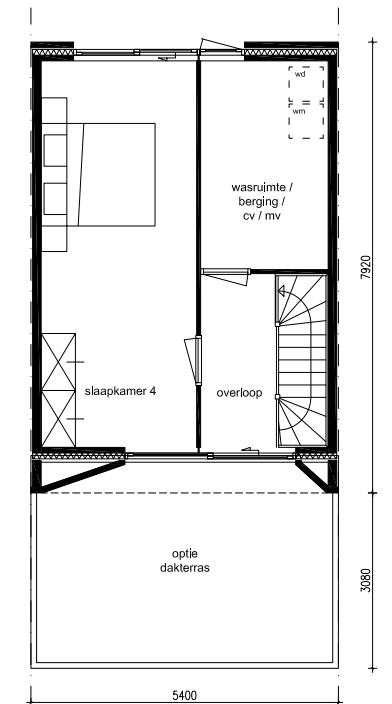
tweede verdieping
