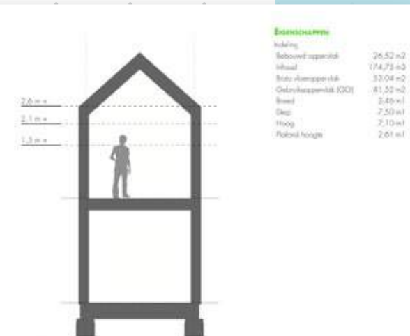
Doorsnede
