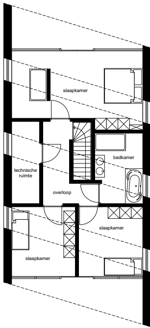
eerste verdieping
