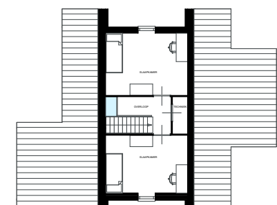
tweede verdieping
