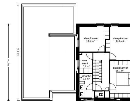
eerste verdieping
