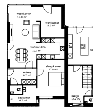
begane grond
