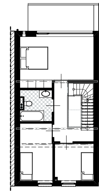
eerste verdieping
