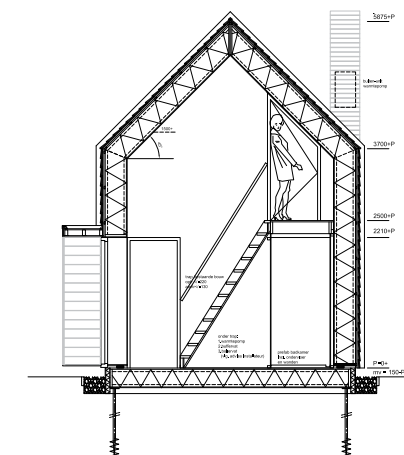
doorsnede
