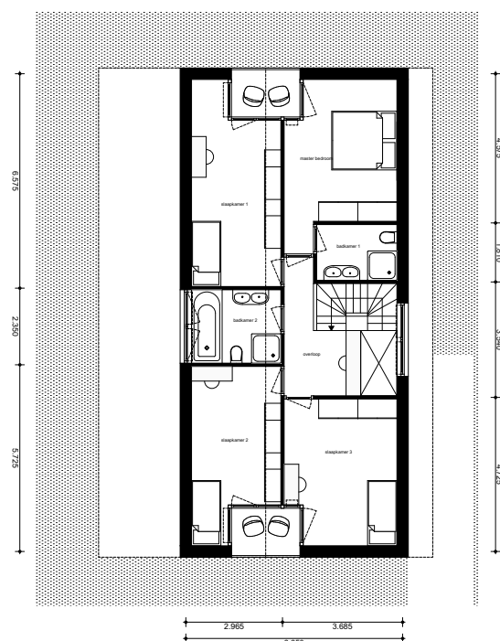
eerste verdieping
