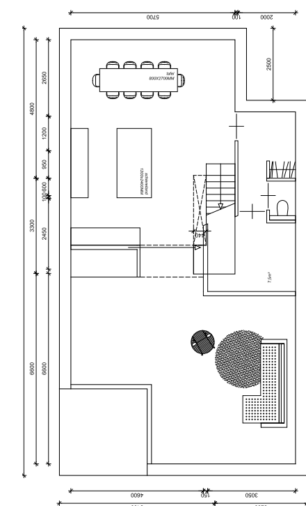
begane grond
